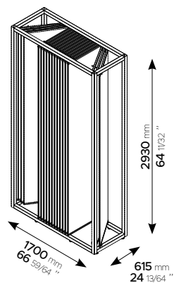
MODULO_FLAG 18+18 _60x280 cm.
