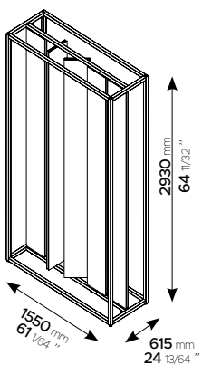
MODULO_SPIN-B 5+5 _30x280 cm.
