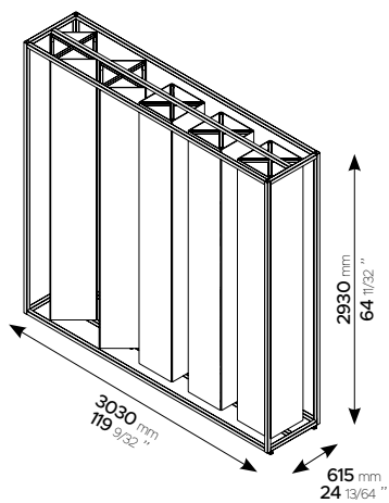
MODULO_SPIN-Q 4x5 _40x280 cm.
