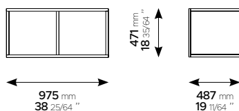
MODULO A GIORNO Open unit Module ouvert Módulo abiertos
